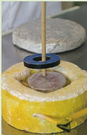
超伝導体の上に浮いている磁石。
